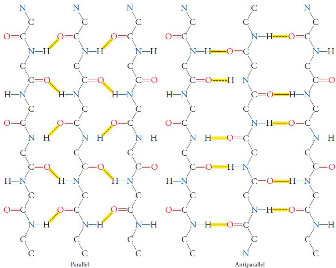
Fig. 3. Feuilletts \beta plissés.
