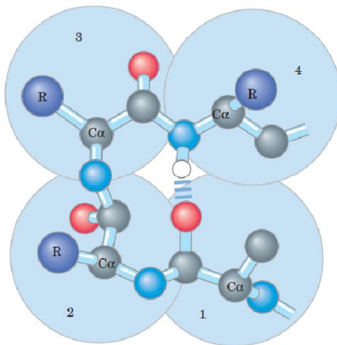
Fig. 4. Coude \beta
