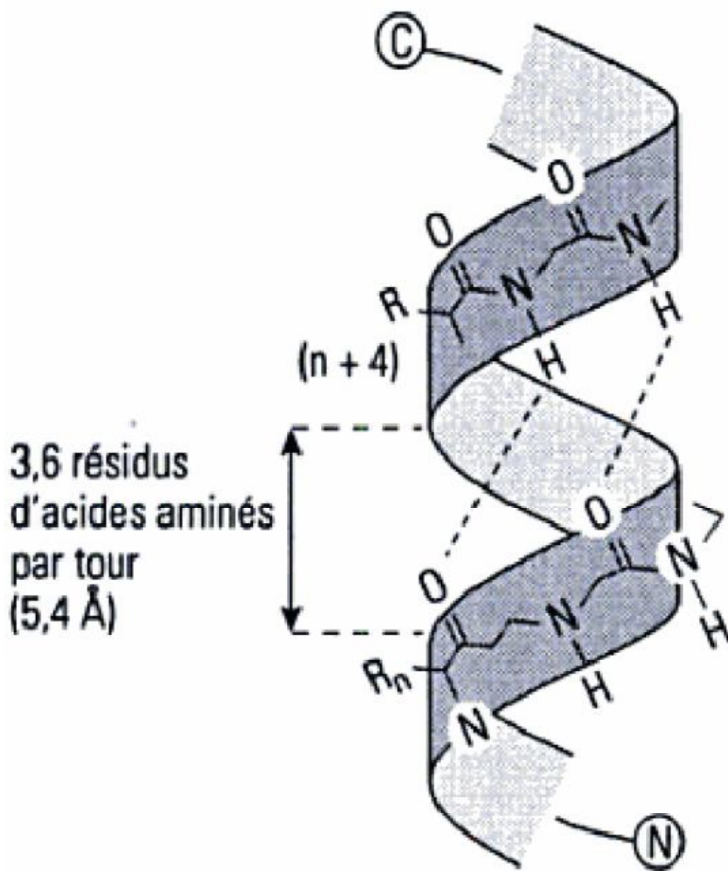
Fig. 2. Hélice \alpha
