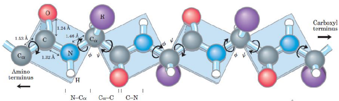
Fig. 1. Particularité de la liaison peptidique.
