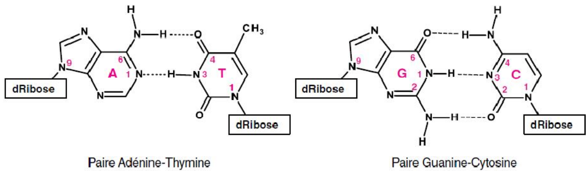
Fig. 6. Liaisons hydrogène entre les bases azotés de l'ADN
