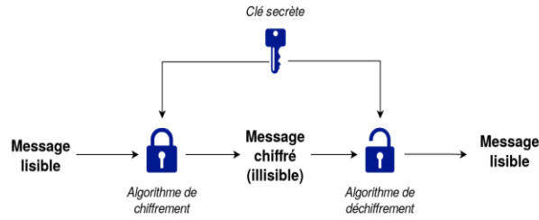
Figure 3.1: Shéma de cryptographie symétrique
