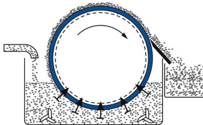
Figure 8 : Filtre rotatif à tambour
