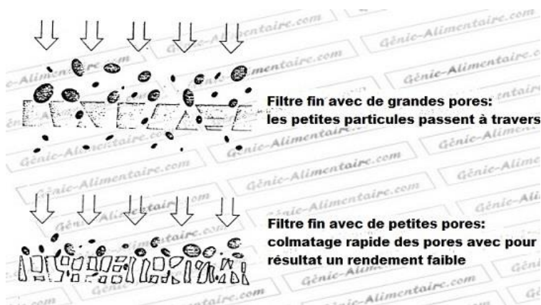
Figure 3 Filtration en surface
