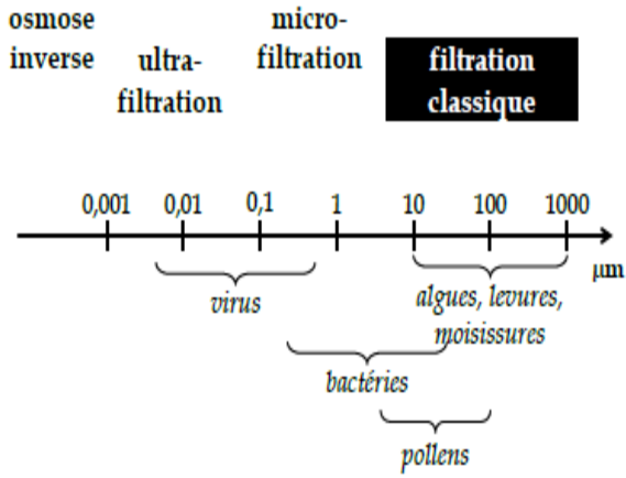
Figure. 1 Catégorie de filtration selon la taille
