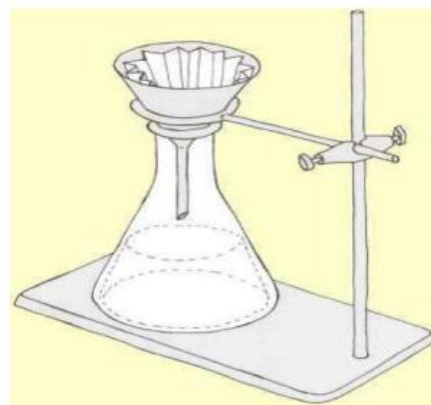
Figure 9 Filtration par gravité
