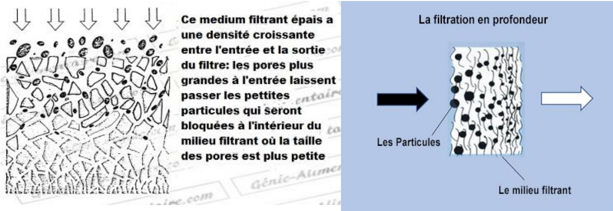
Figure 4 Filtration en profondeur
