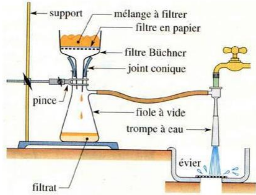
Figure 10 Filtration sous vide
