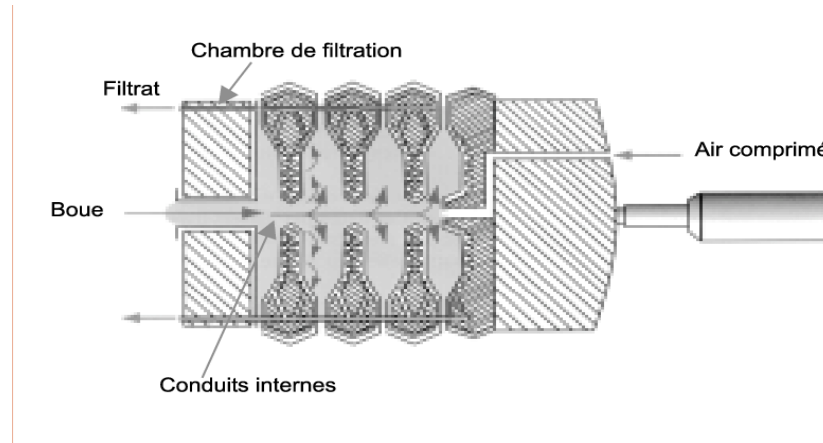
Figure 7 : Filtre presse à plateaux
