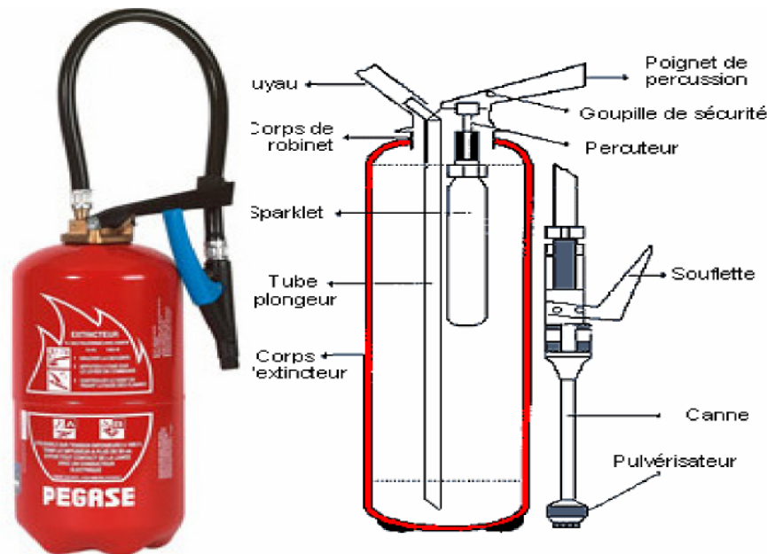
Figure IX.12 : L'extincteur
