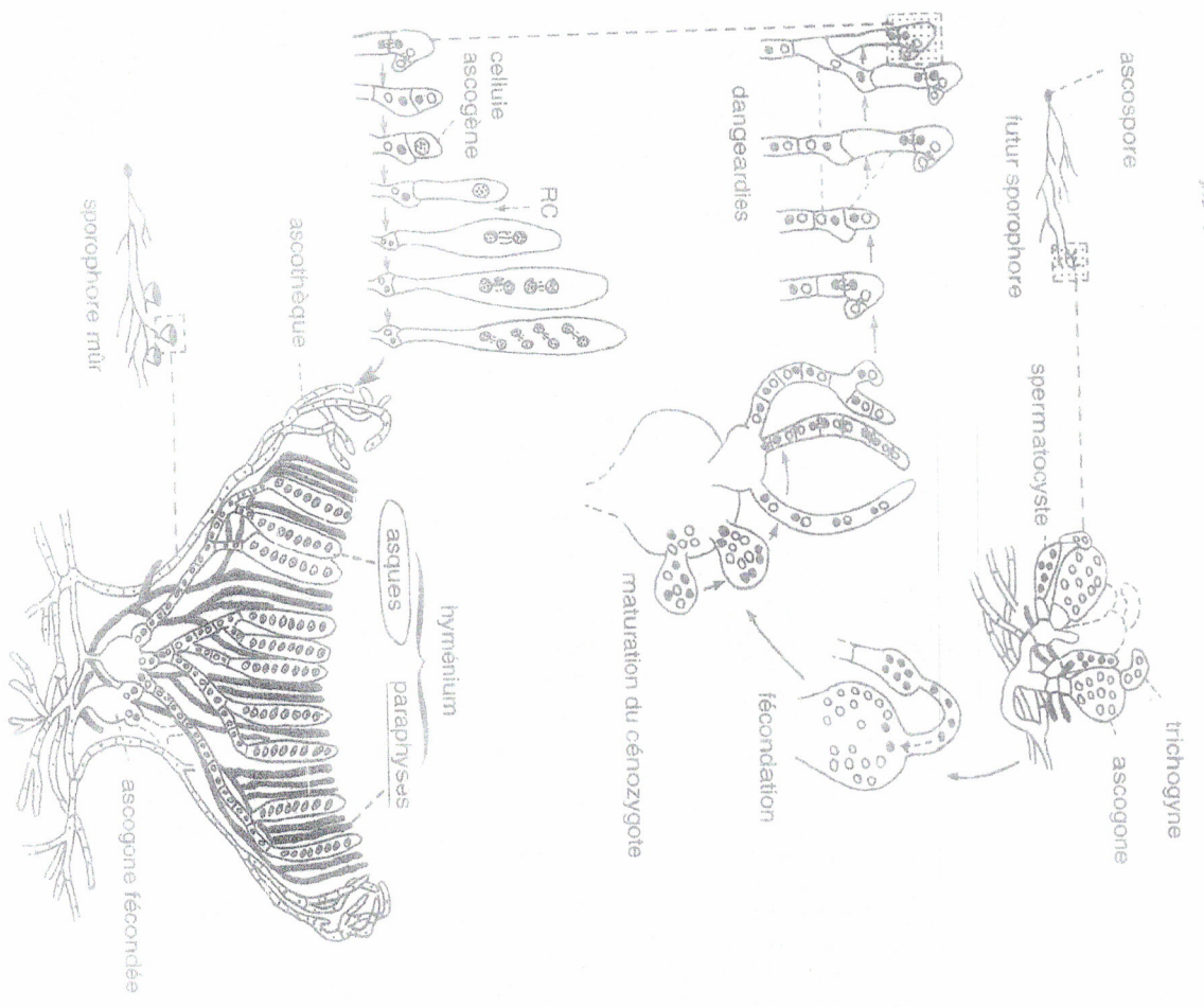
Fig. 5.3. Cycle de développement de Pyrenopeziza omphalodes .
