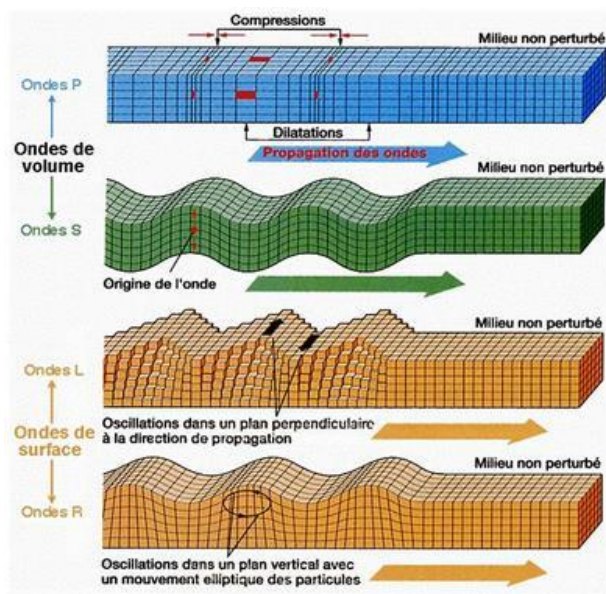
Fig. 36 Les différents types d ondes
