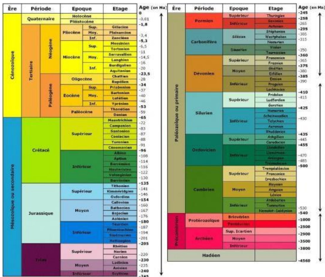
Fig. 25 Echelle stratigraphique
