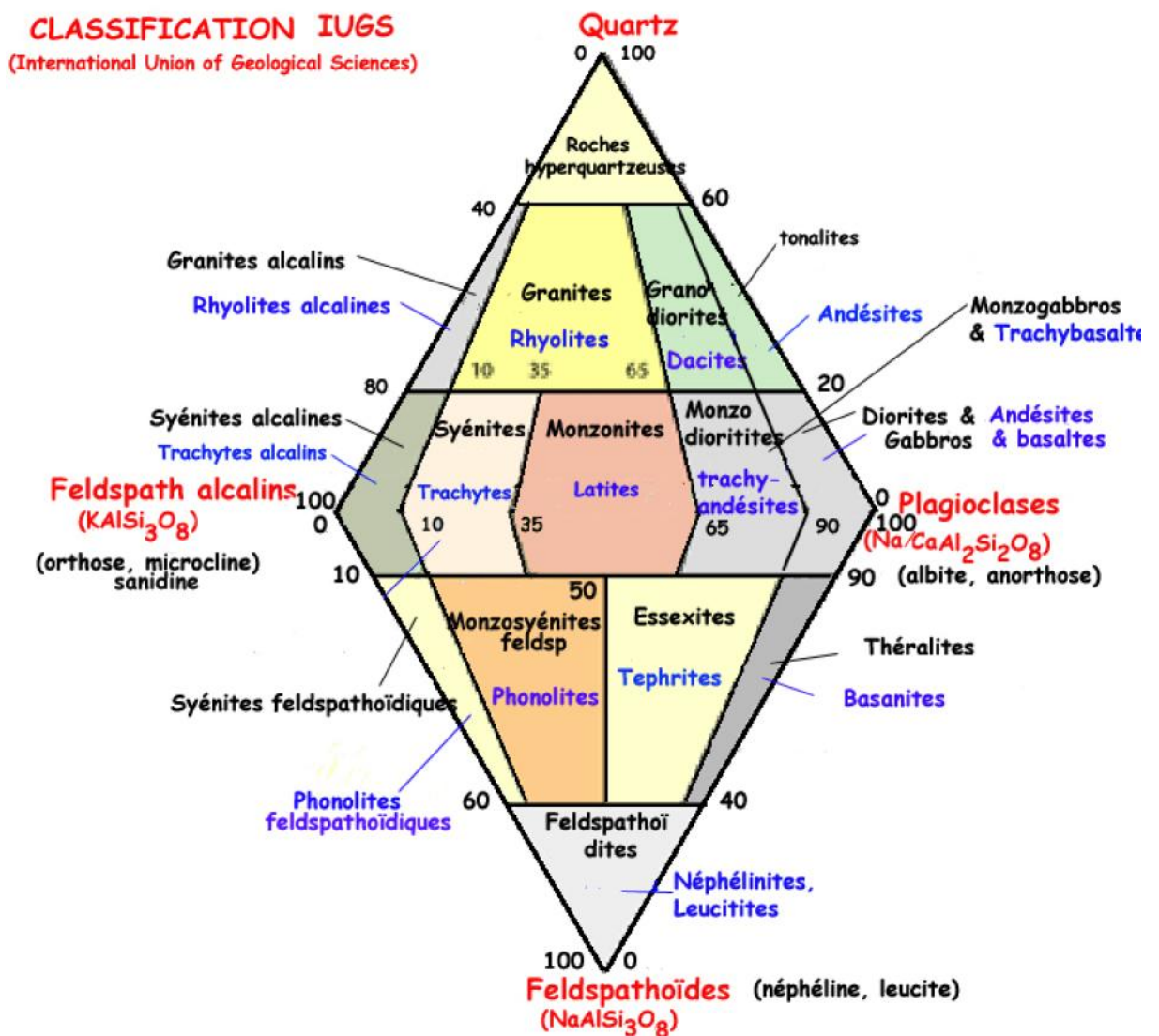
Fig. 46 classification de Streckeisen
