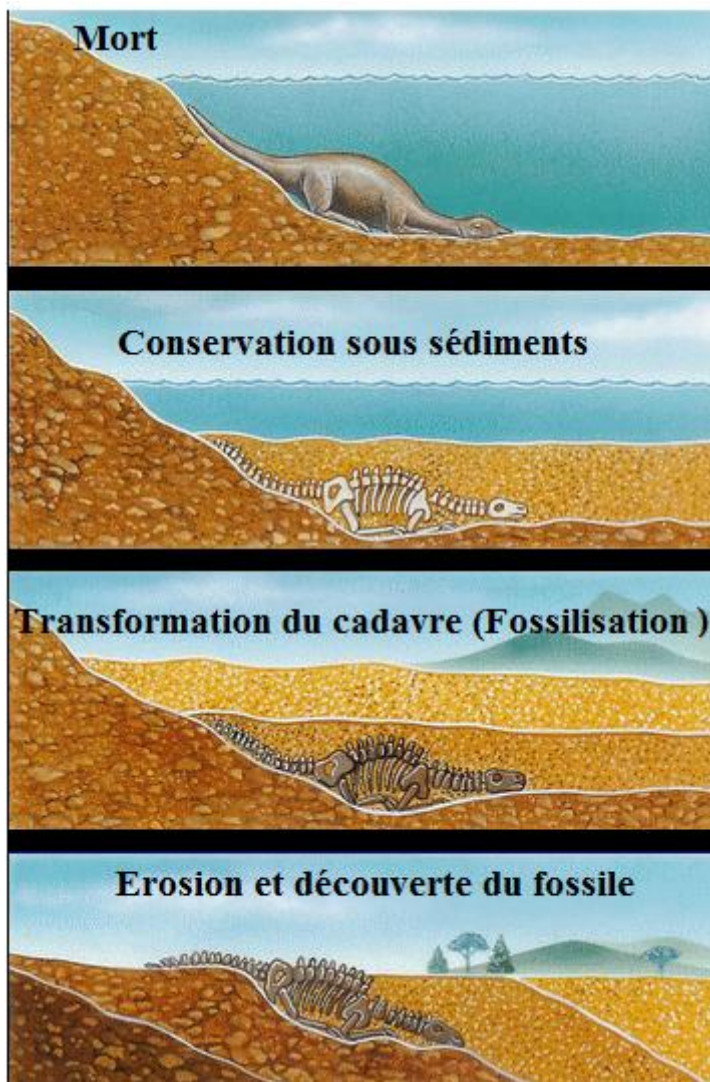
Fig. 26 Les étapes de la fossilisation
