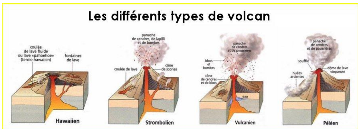
Fig. 42 Les différents types de volcans
