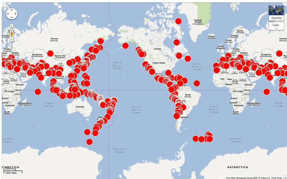
Fig. 40 Répartition des Séismes
