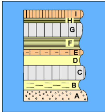
Fig. 18 Principe de superposition
