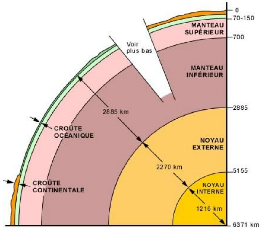
Fig.7 Structure interne de la terre (u.laval.can )
