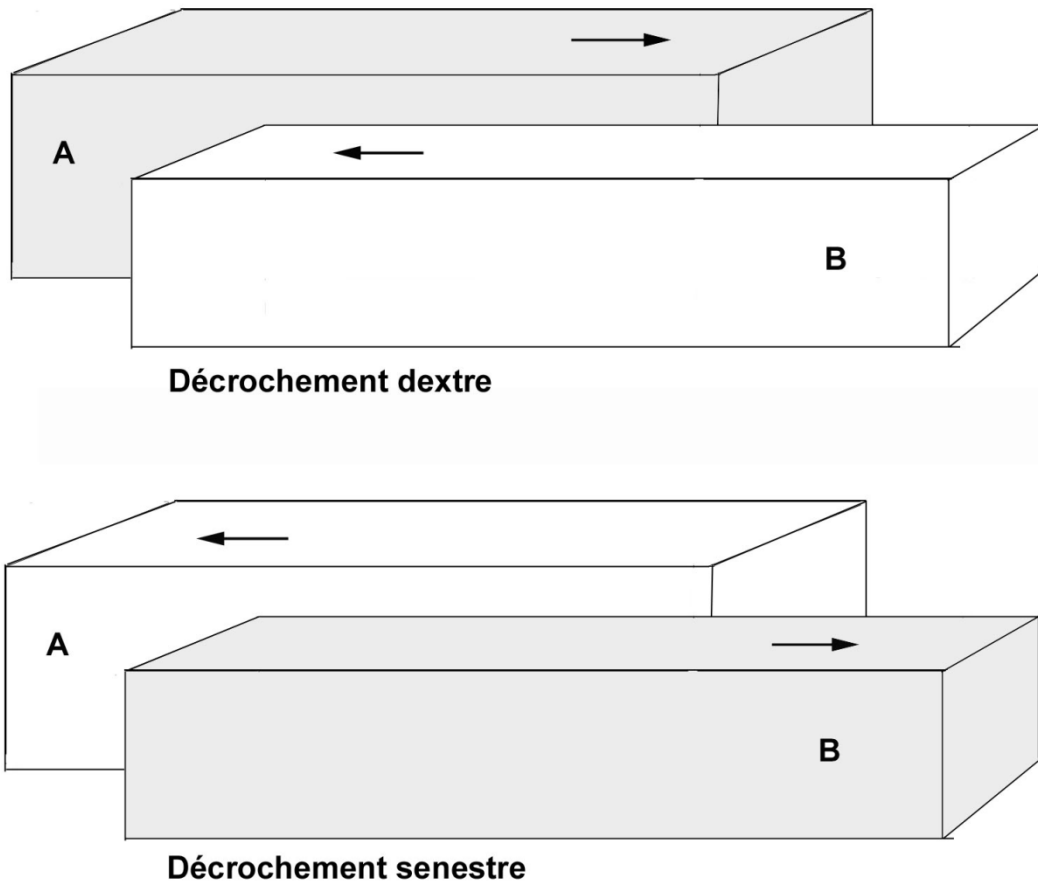
Fig. 31 Décrochements dextre et senestre
