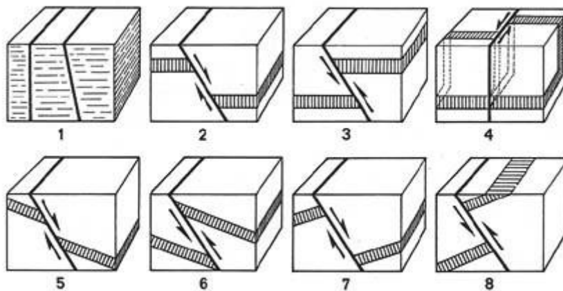
Fig. 29 Types de failles : 1 – failles verticales et obliques ; 2 – faille normale ; 3 – faille inverse ; 4 – décrochement ; 5 – faille conforme normale ; 6 – faille conforme inverse ; 7 – faille contraire normale ; 8 – faille contraire inverse (Foucault A. & Raoult J.F. 1975).
