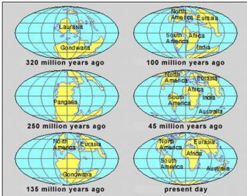
Fig. 52 Evolution de la théorie de Wegener
