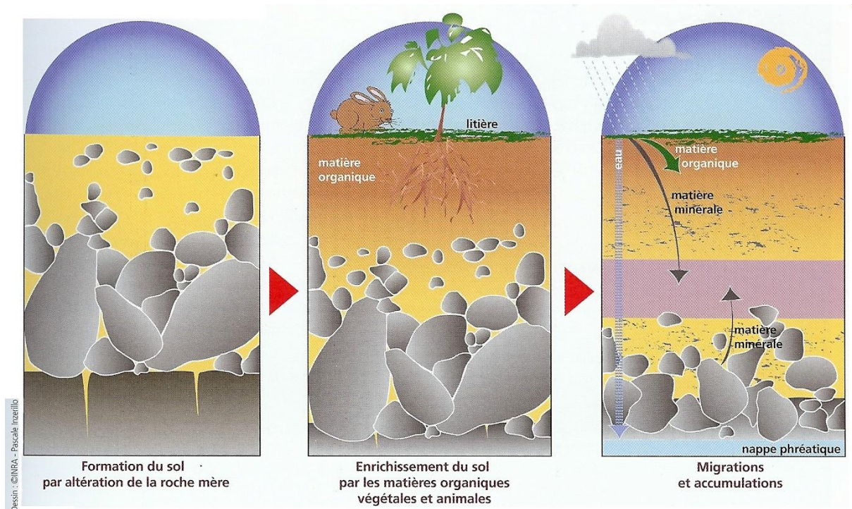
Fig. 16 Mode de formation du sol
