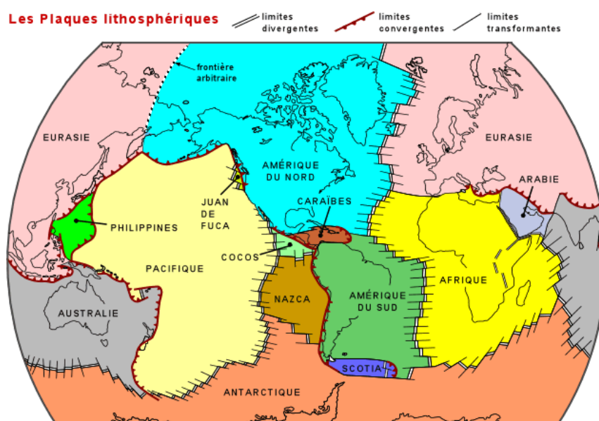
Fig 50 Les palques tectoniques
