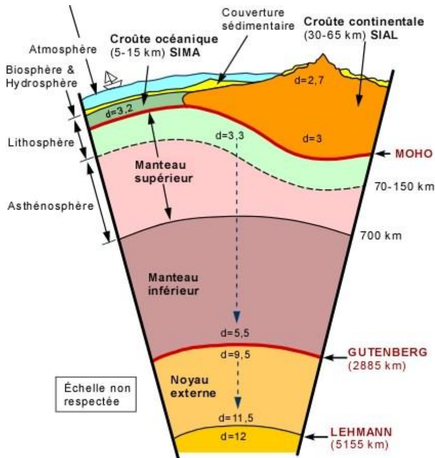
Fig. 8 Les différentes discontinuités de la terre (univ.laval.can )
