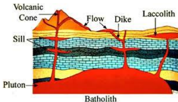
Fig.43 Modes de gisement des roches magmatiques
