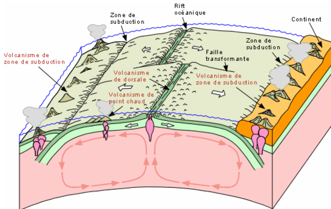
Fig. 51a Limites entre les plaques
