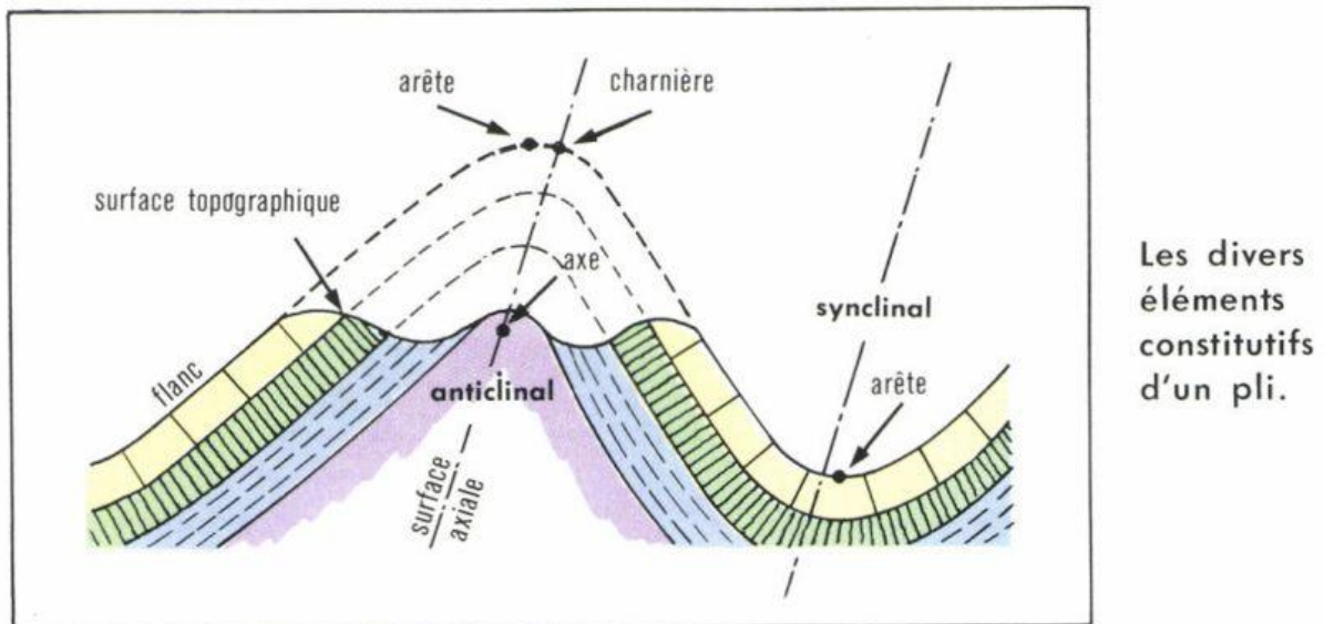
Fig. 33 Les éléments d'un pli
