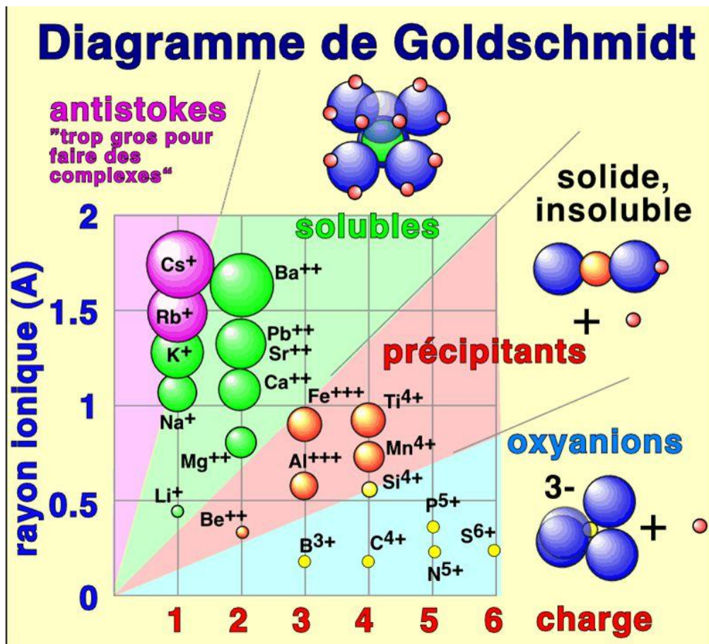
Fig. 11 Diagramme de Goldschmidt
