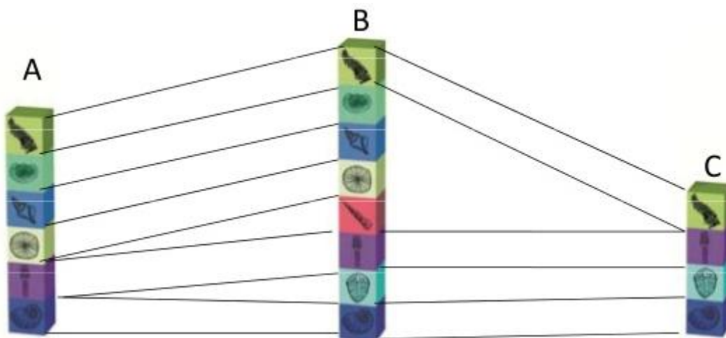
Fig. 22 Corrélation des couches en même contenu fossilifère
