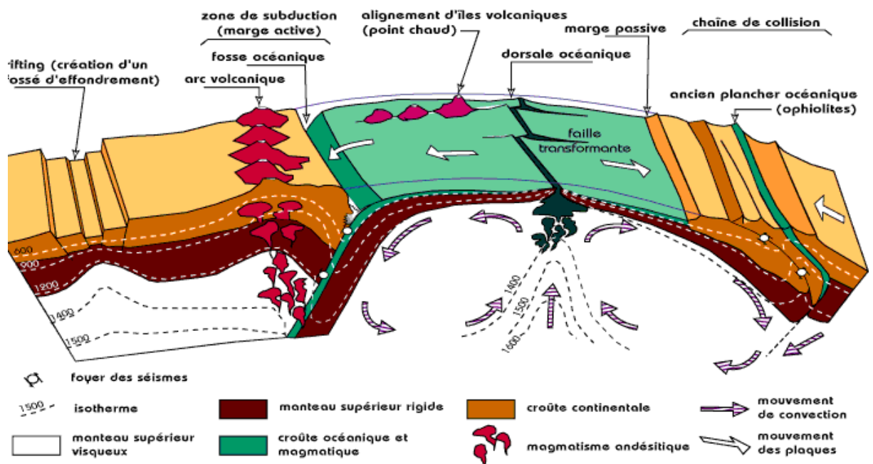
Fig. 53 Théorie de la tectonique des plaques
