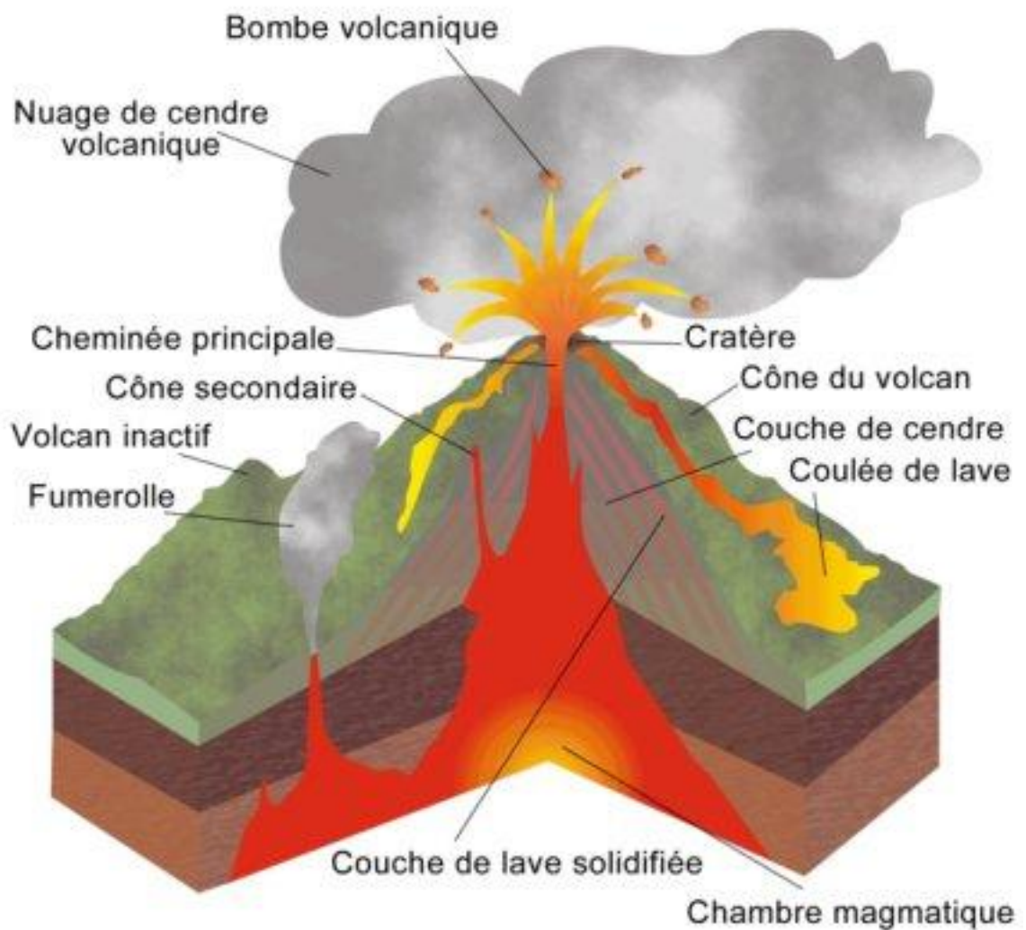
Fig. 41 Schéma d'un Volcan
