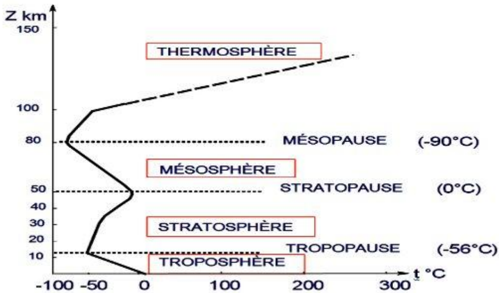
Fig. 2 Les enveloppes de l'atmosphère (Météo France éducation)
