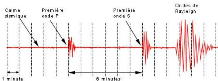
Fig. 39 Sismogramme
