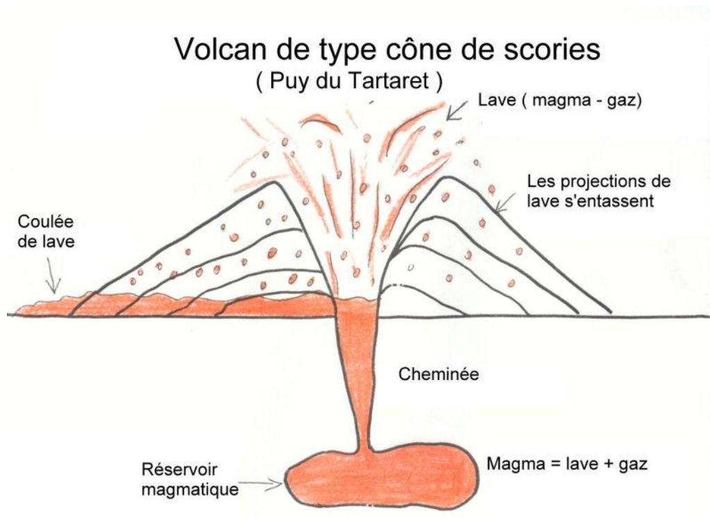
Fig. 44 Projection d'un volcan
