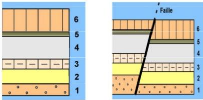
Fig. 20 Principe de recouplement
