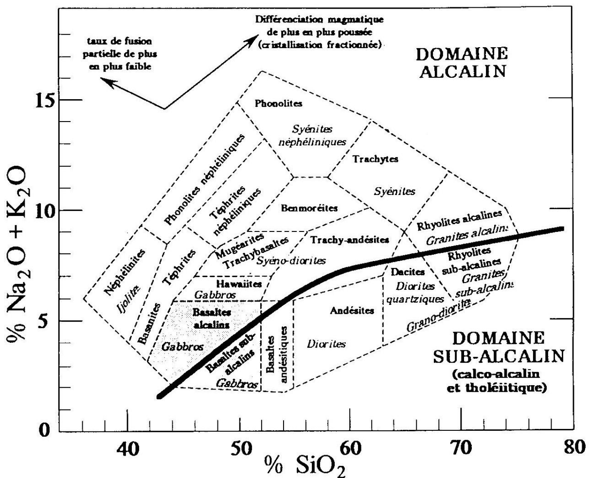
Fig. 47 classification chimique des roches magmatiques
