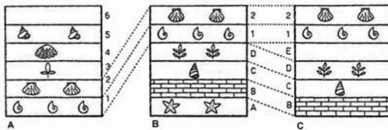
Fig. 19 Principe de continuité
