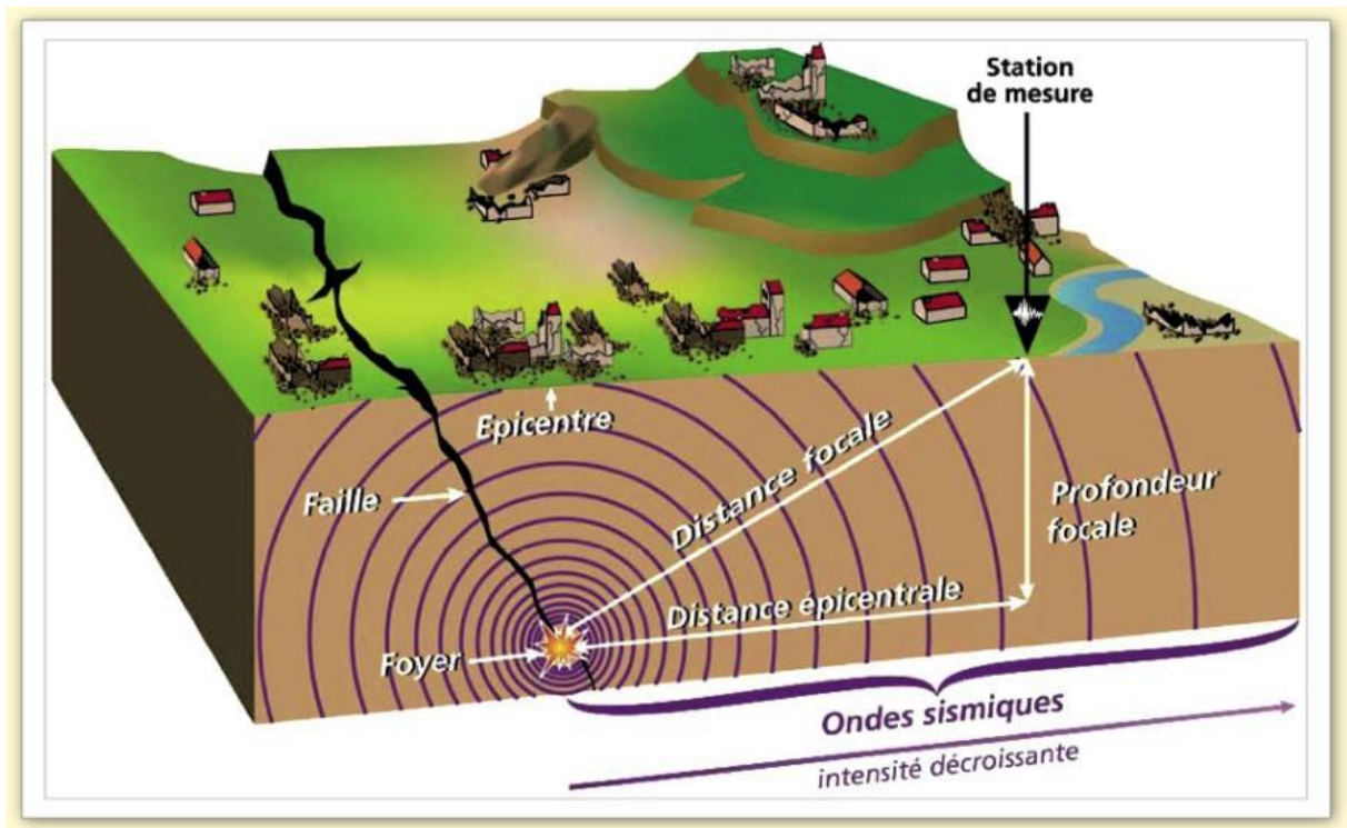
Fig. 35 Foyer d un Séisme
