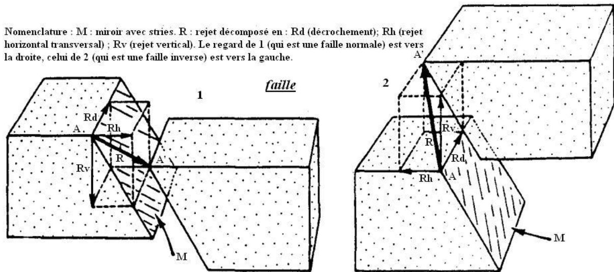
Fig. 28 Les éléments d'une faille (Mattauer 1973)
