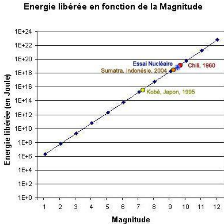
Fig. 37 Echelle de Richter
