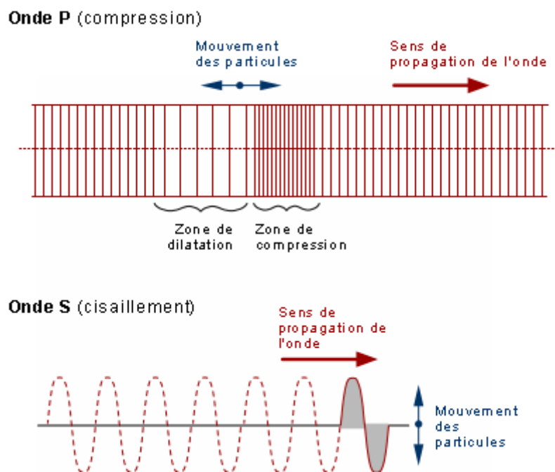
Fig. 9 Les ondes de volumes
