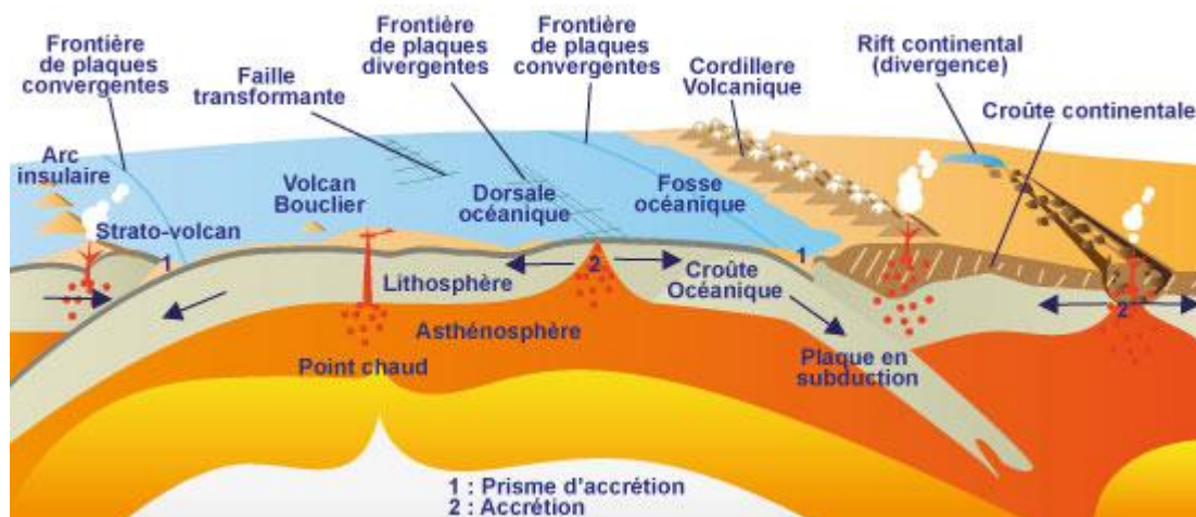
Fig. 52b Les différentes frontières
