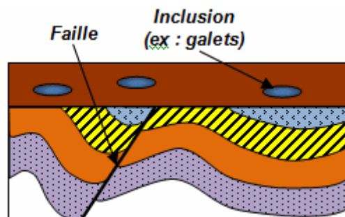
Fig21 Principe d'Inclusion
