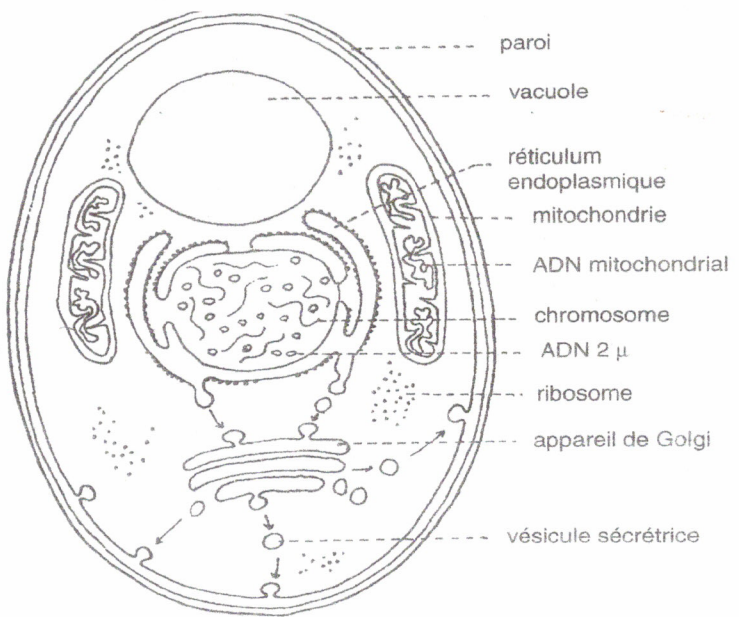
Fig. 9.12. Schéma de l'ultrastructure de Saccharomyces cerevisiae .
