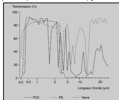
Figure 1-11. Spectre de transmission de quelques substances (PVC = chlorure de polyvinyle, PE = polyéthylène).
