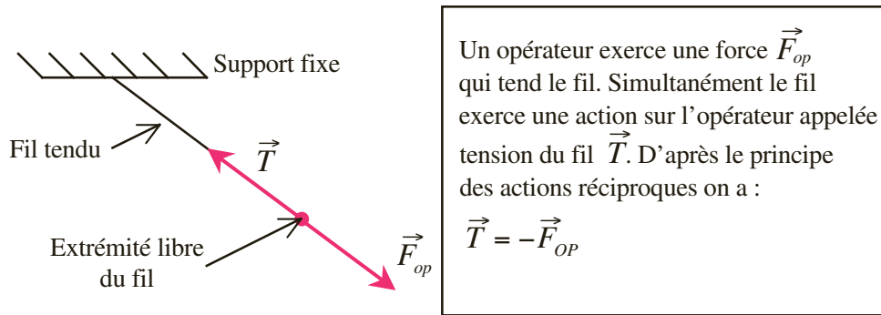
Figure 2.12 Tension d'un fil.
