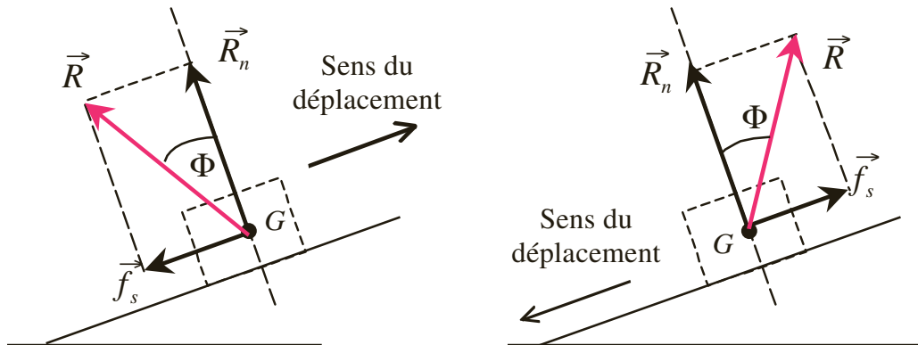
Figure 2.11 Représentation de la force de frottement solide f_s suivant le sens du déplacement de G . Les autres forces appliquées sur G ne sont pas représentées.
