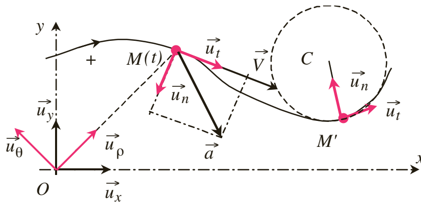
Figure 1.18 Le vecteur accélération et la base de Frenet ( \vec{u}_t, \vec{u}_n ). Le rayon de courbure en M' correspond au rayon CM' du cercle tangent à la trajectoire au point M' considéré. Les bases polaire et cartésienne sont représentées au point O pour mettre en évidence les différences avec la base de Frenet.
