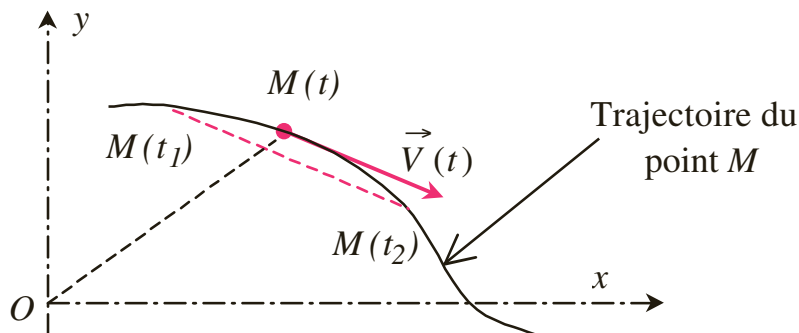
Figure 1.11 Vecteur vitesse \vec{V}(t) tangent à la trajectoire au point M(t) considéré.
