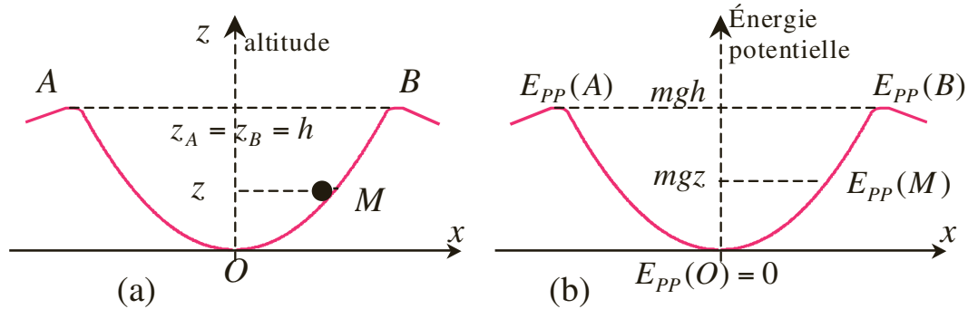
Figure 3.9 Le graphe (a) représente le profil du sol (altitude z ) en fonction d'une abscisse x . Le graphe (b) représente l'énergie potentielle en fonction de la position.
