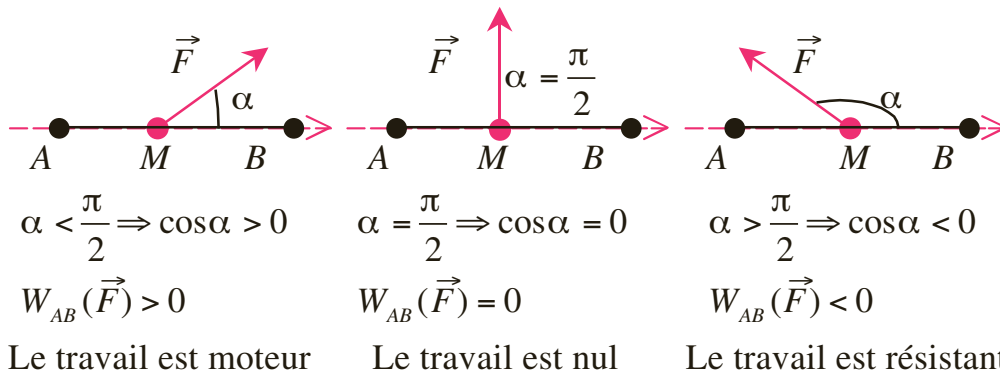
Figure 3.2 Travail moteur, nul et résistant d'une force.
