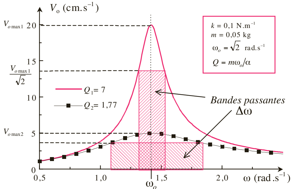
Figure 5.7 Bandes passantes en hachuré pour deux amortissements différents.
