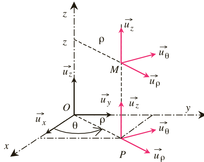
Figure 1.7 Le système de coordonnées cylindriques.
