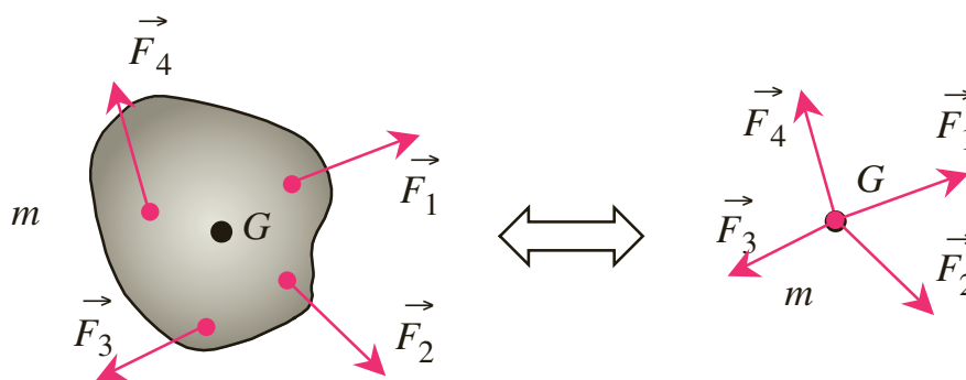
Figure 2.5 Illustration du théorème du centre d'inertie.
