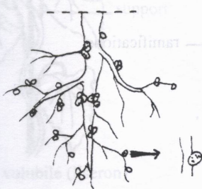
Figure 5: nodosités (racine + bactérie).
