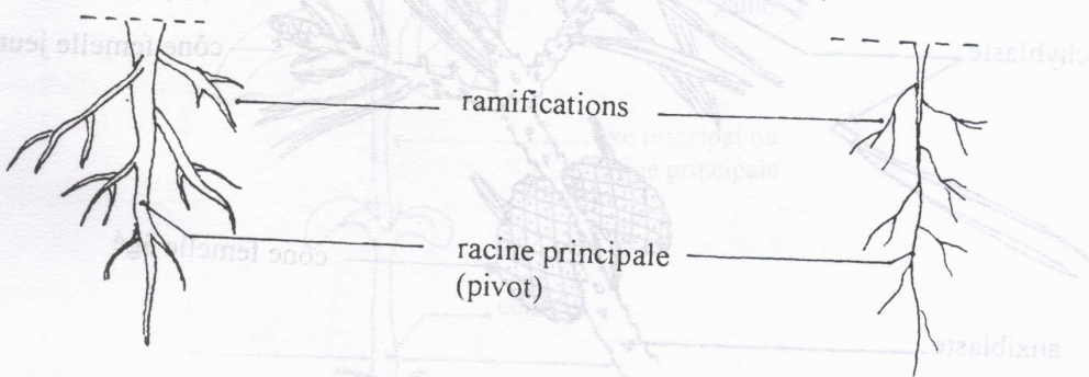
Figure 3 : Systèmes racinaires pivotants .
