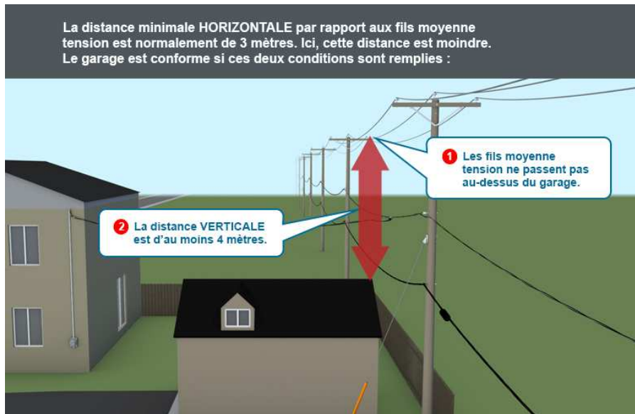
Figure VIII.6 : Exemple illustré - Ajout d'un garage à moins de 3 mètres d'une ligne de distribution
