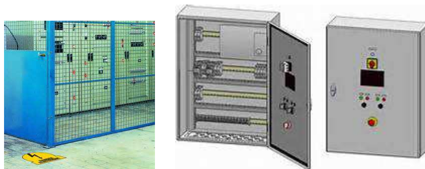
Figure VII.11 : Protections permanentes par Grillage (a) et porte (b) d'armoire électrique
