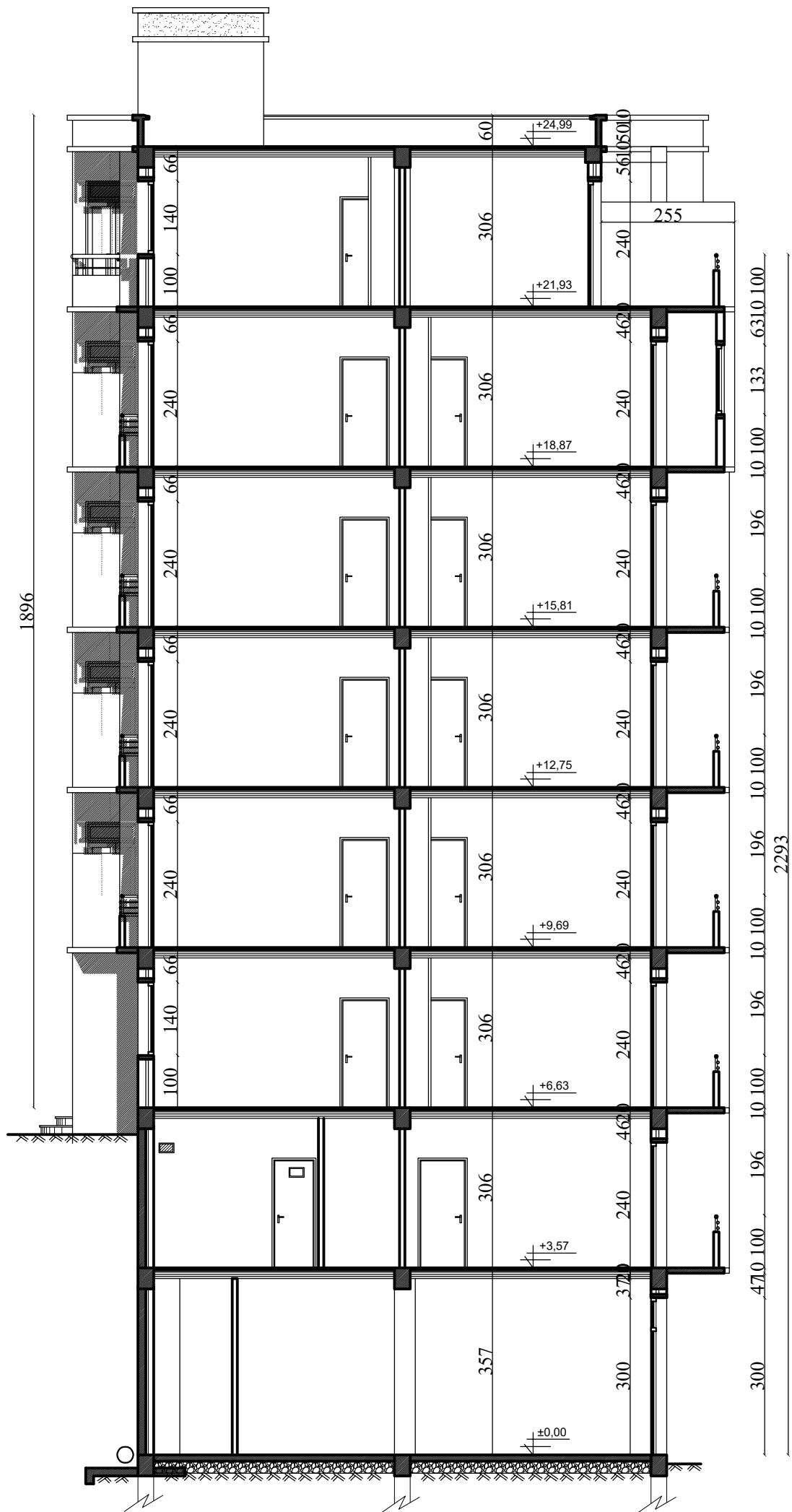
COUPE B-B
