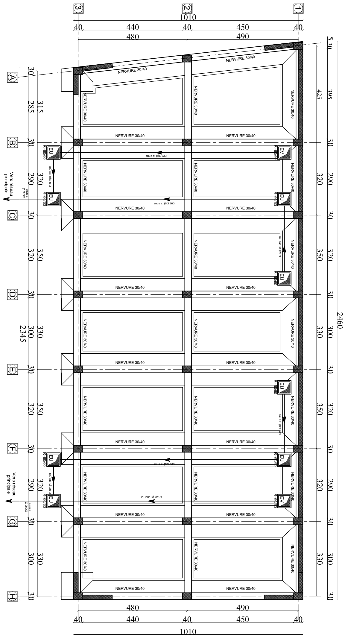
PLAN DE FONDATION
